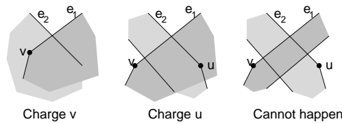
Fig. 142: Proof of Lemma 2.
